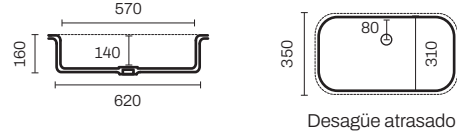
Desagüe atrasado
